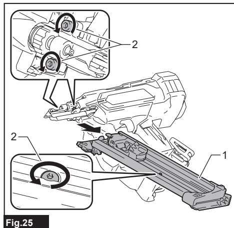
Fig. 25 ► 1. Magazine 2. Bolts
